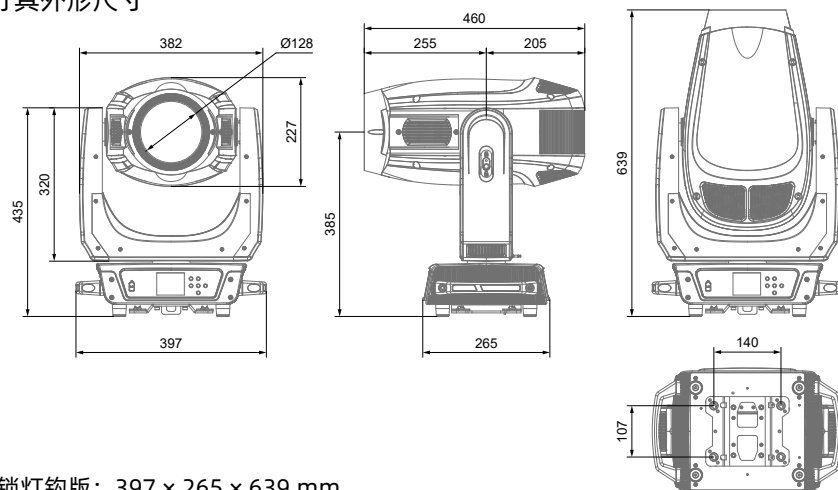
快锁灯钩版：397 × 265 × 639 mm
