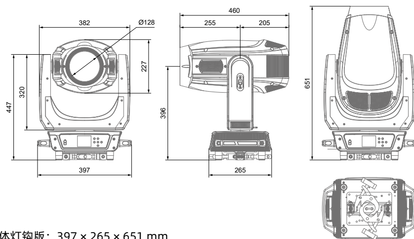
一体灯钩版：397 × 265 × 651 mm
