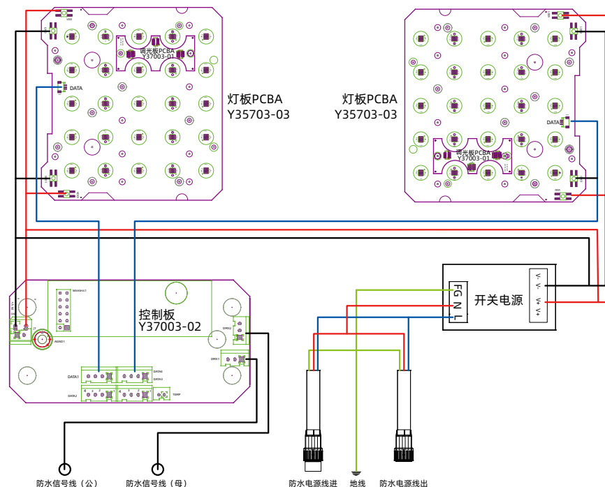
九、控制线路图
