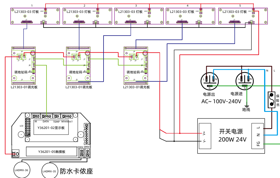
九、控制线路图
